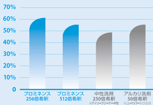
▶ JFPA洗浄力比較試験結果
